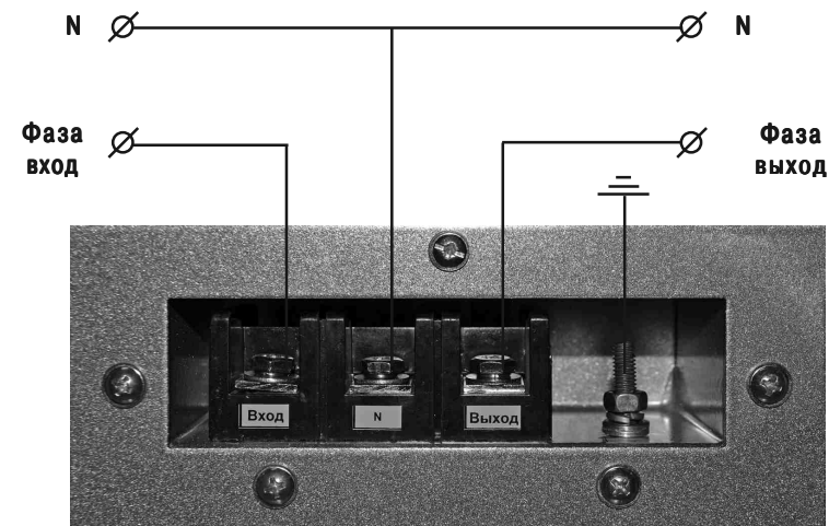
Рис. 3. Схема подключения стабилизатора
